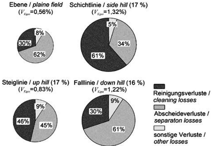
Abb. 1: Kornverluste am Mähdrescher nach BÖTTINGER, FLIEGE, (Quelle: LANDTECHNIK online 1.2012)
